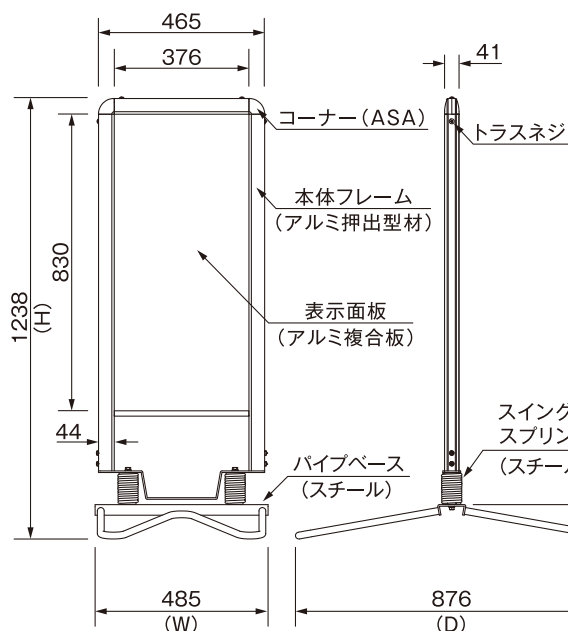
寸法図
